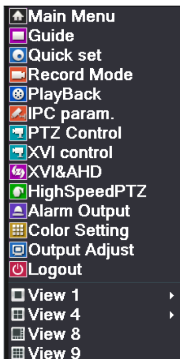
Shortcut Menu
